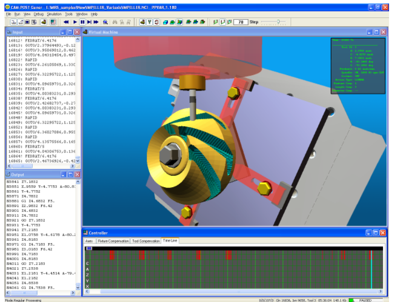
ポスト処理実行中にホルダー干渉、固定具干渉を検出
