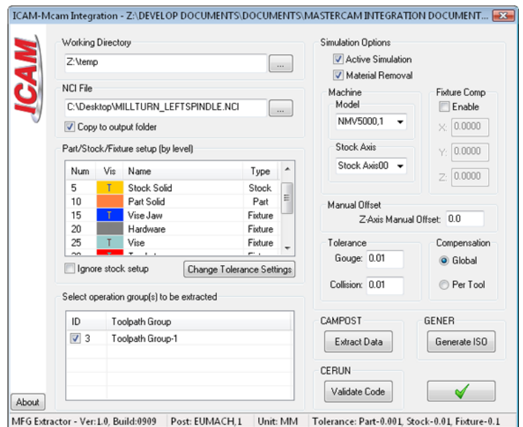
Mastercam 専用の加工情報抽出画面
